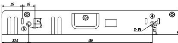
前视图
