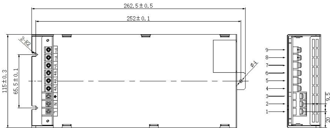
端子脚位定义
