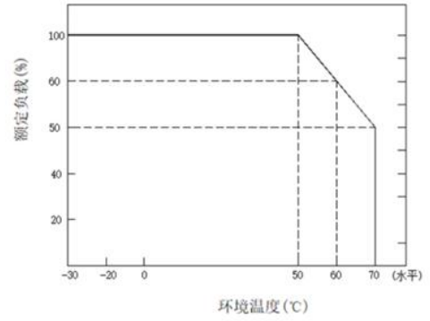
输出负载与温度曲线 (36V 48V)
