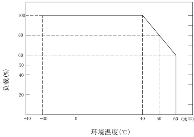
环境温度与负载降额曲线 (36V)
