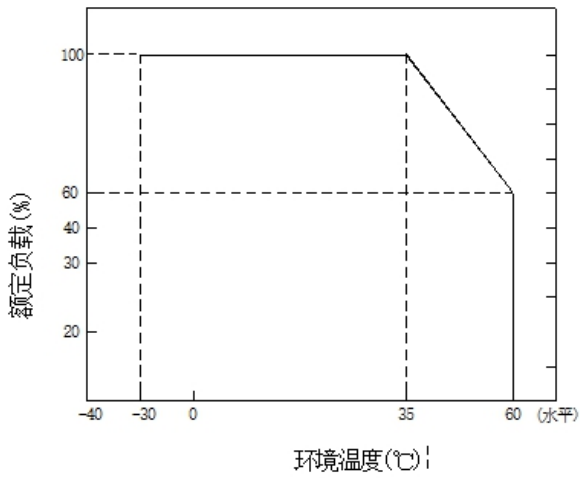
环境温度与负载降额曲线 (36V)
